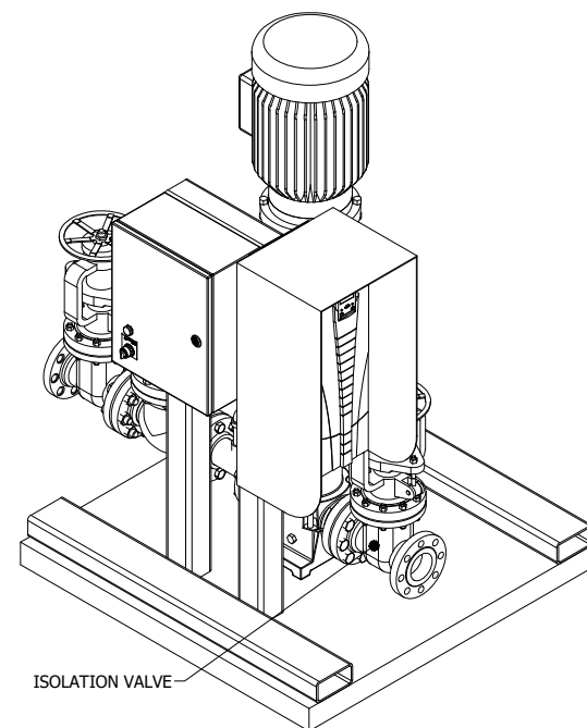
ISO BACK RIGHT (SUCTION SIDE)
